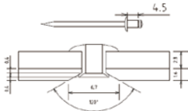
母材板厚 t2.3+t1.6の場合
