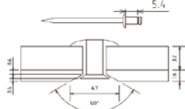
母材板厚 t3.2+t1.6の場合
