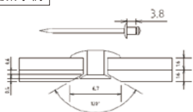
母材板厚 t1.6+t1.6の場合
